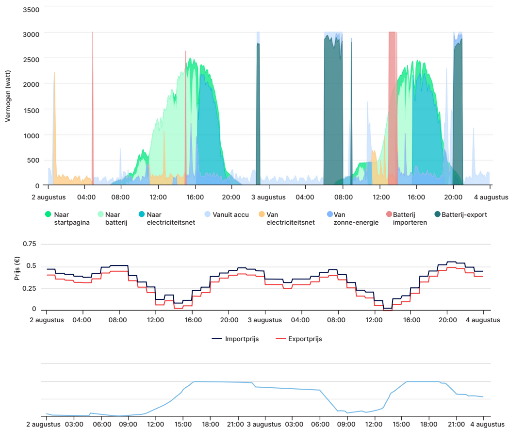
SolarEdge ONE batterijoptimalisatie in een residentiële site in Nederland, wat een dynamisch tarief aantoont.
